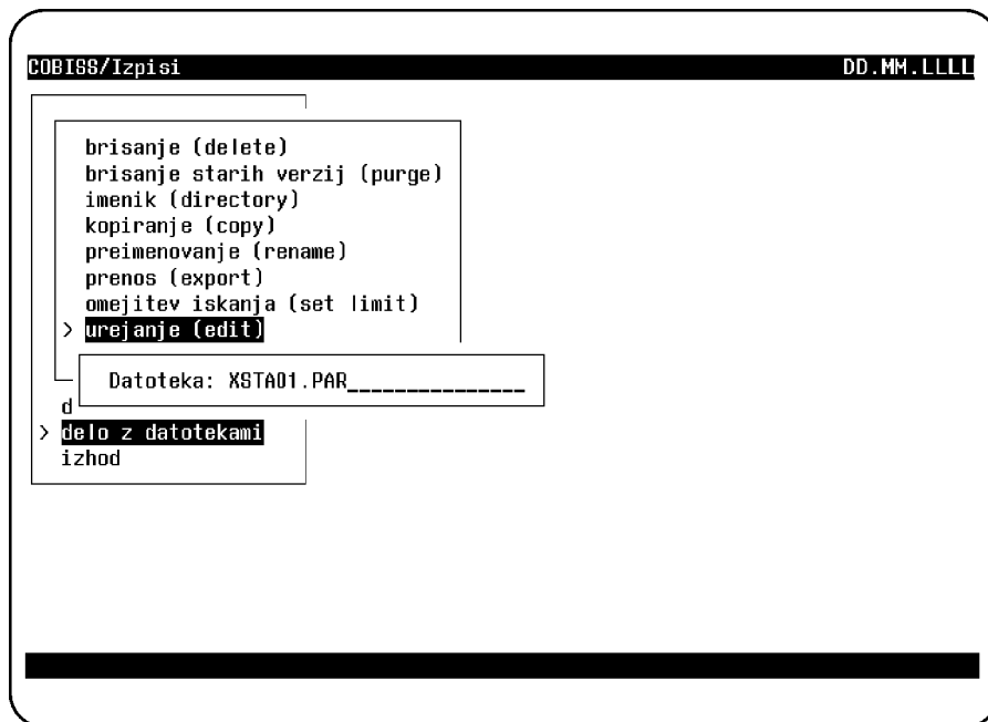
Slika 3.8 - 1: Uređivanje datoteke
