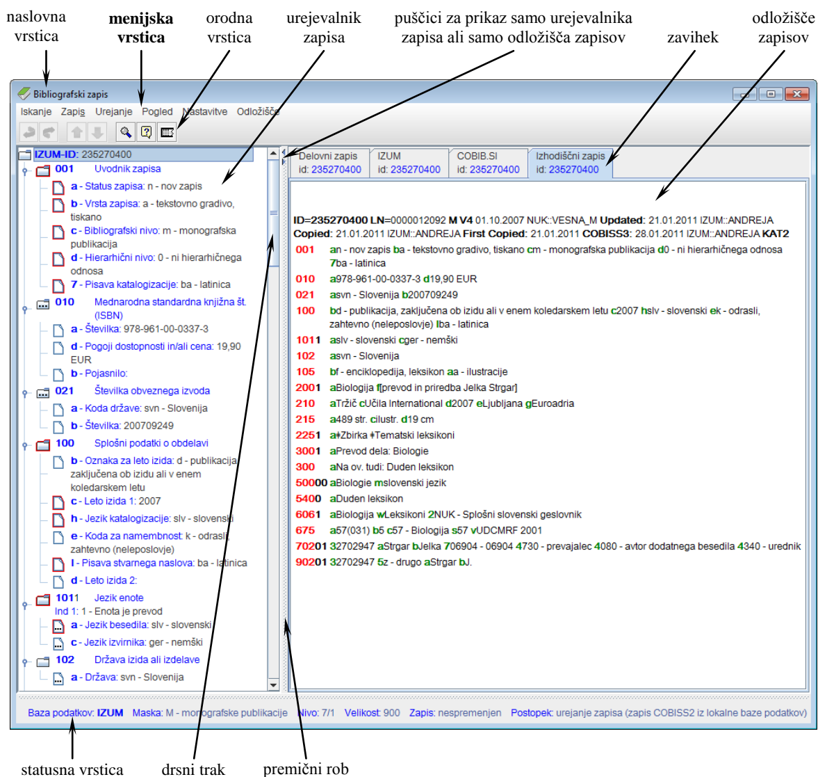
Slika 3-2: Vmesnik za katalogizacijo
