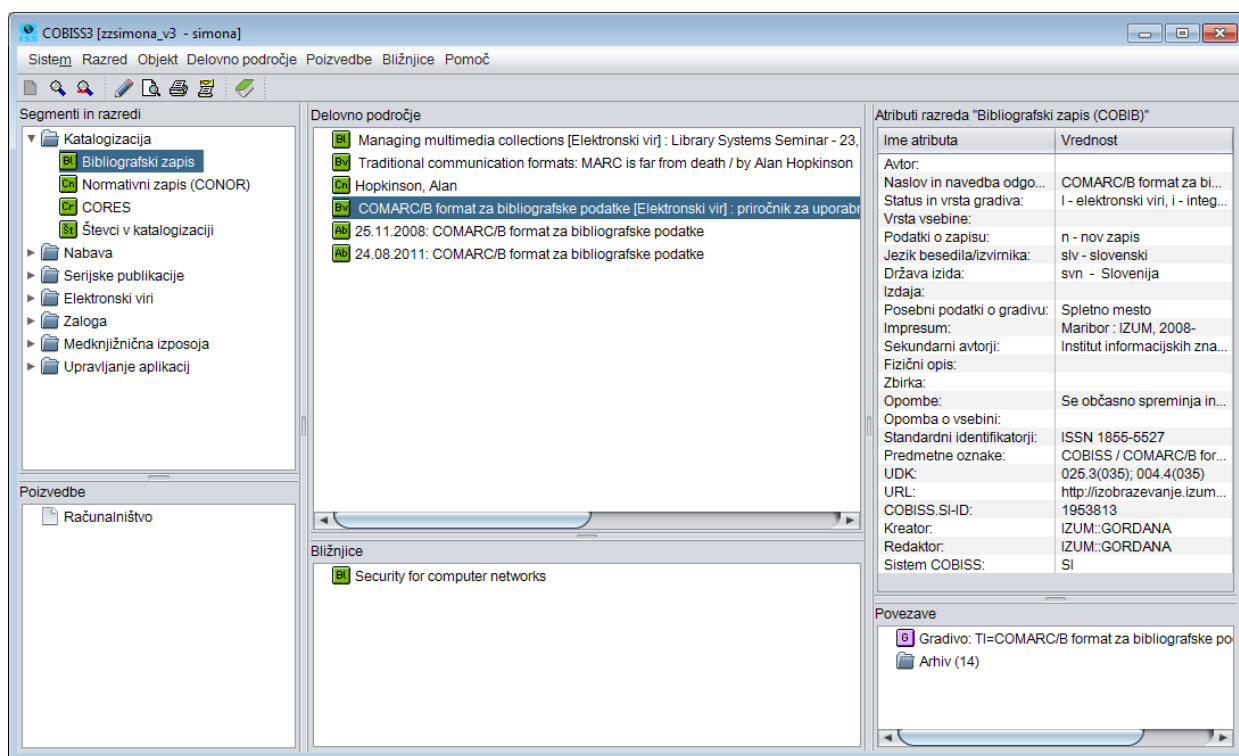
Slika 11-1: Brskalnik – podokna
